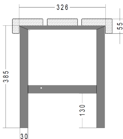
TUBE ROND, variante avec grille à chaussures rabattable
