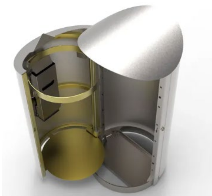
Cleveres Innenleben für einfaches Wechseln der Abfallsäcke
